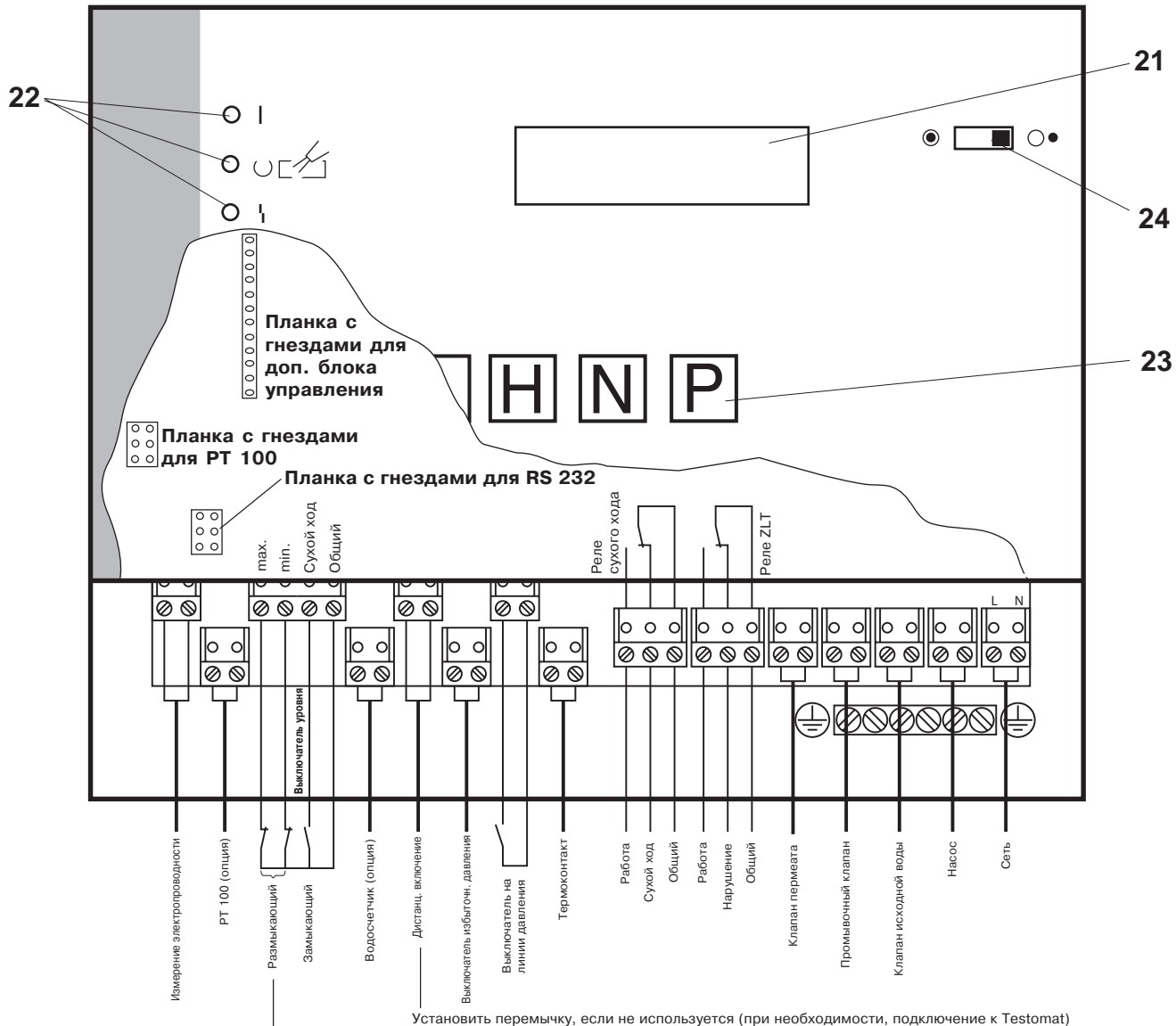
Рис. 1: Схема включения Если нет выключателя уровня, установить перемычку между "макс." и "общий"
